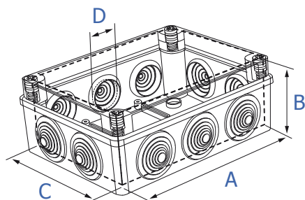
Wymiary A, B, C są wymiarami wewnętrznymi S-BOX Dimensions A, B, C - dimension inside S-BOX
