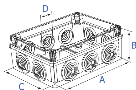
Wymiary A, B, C są wymiarami wewnętrznymi Dimensions A, B, C - dimension inside
